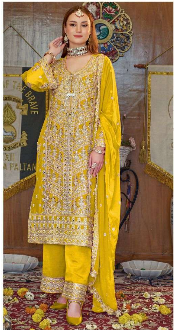
CN-318 B
